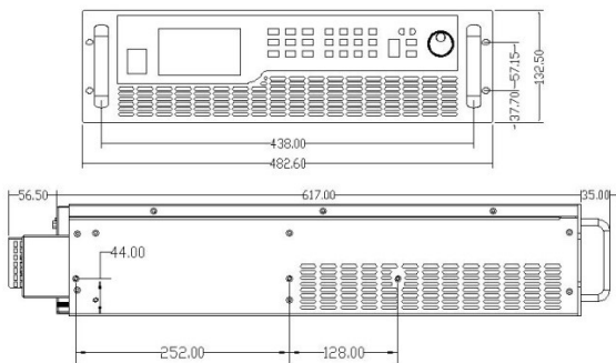
5kW~15kW机型尺寸图（40V以下机型）
