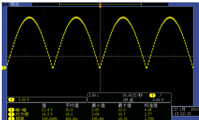
序列功能生成的半波正弦
