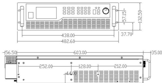
5kW~15kW机型尺寸图（40V及以上机型）
